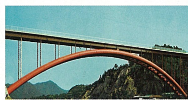
松島橋
